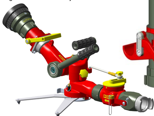
Monitor Poket con oscilador, dispositivo de seguridad anti-oscilación y válvula 1/4
