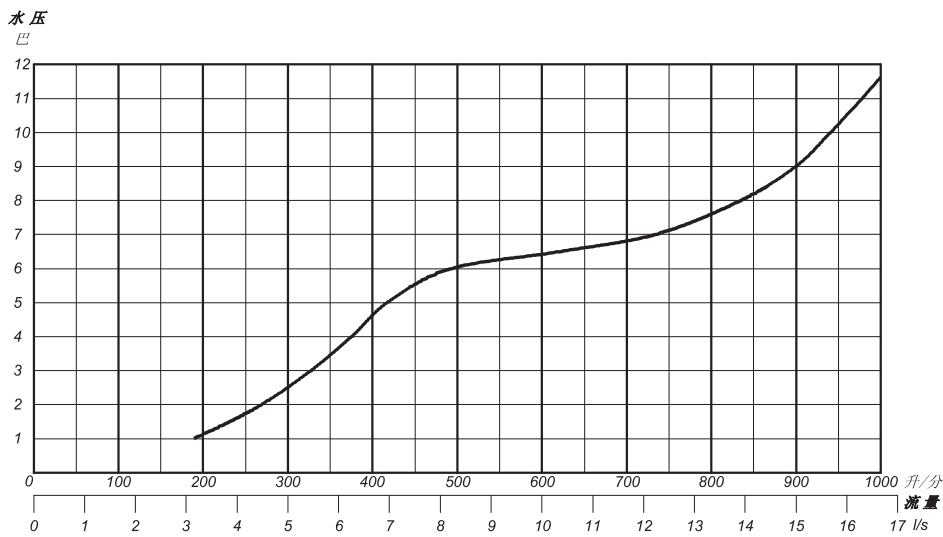
« 诺曼 500 北京式 » 水压和流量关系图
